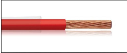
THHN / THWN | 600V
